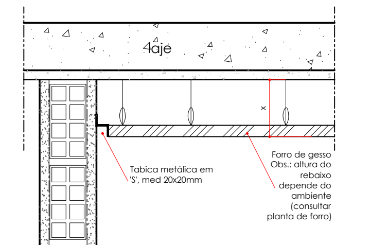
DETAILHE 01 ESC.: 1:10
