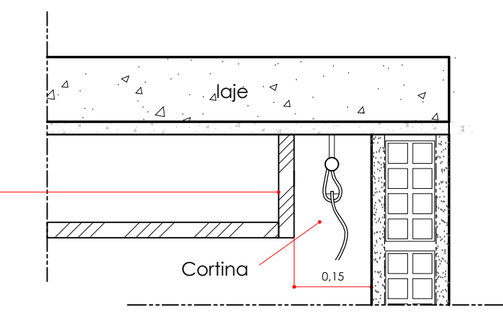
DETAILHE 04 ESC.: 1:10
