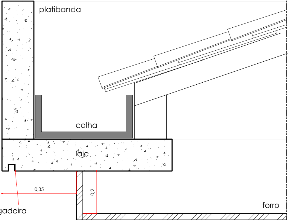
DETAILHE 02 ESC.: 1:10
