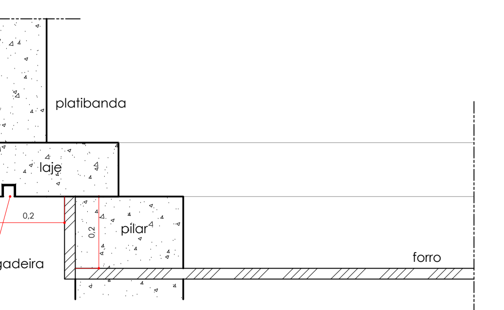
DETAILHE 03 ESC.: 1:10
